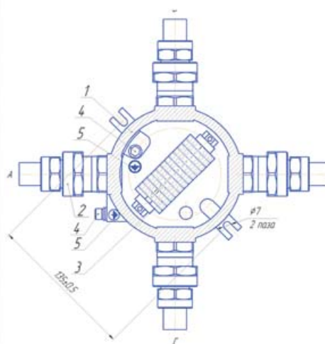
1-корпус, 2-обод кабельный, 3-клеммник, 4-зажим заземления 5- знак заземления
