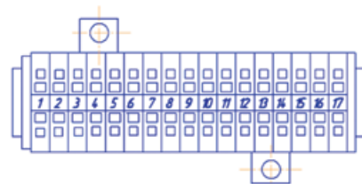
Клеммник 864.04.00.00 (1)- (до 6 шт. в коробке) с клеммами WAGO (тип - 00)
