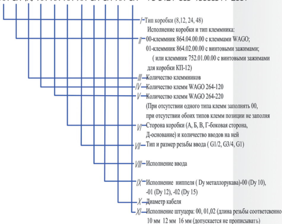
Рисунок 1 - Схема условного обозначения коробки соединительной типа КП
