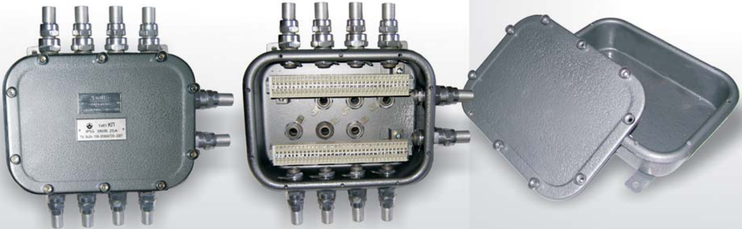
Комплект КП-48 (корпус + крышка)
