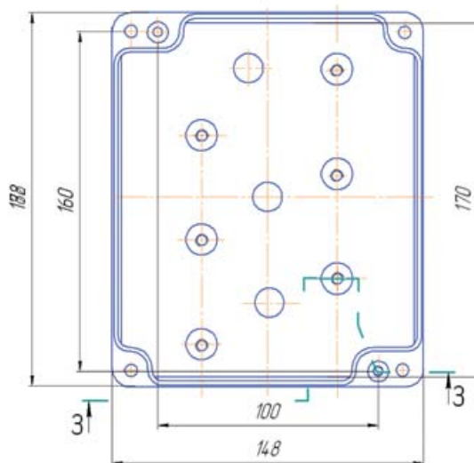
Рисунок - Габаритные и присоединительные размеры
