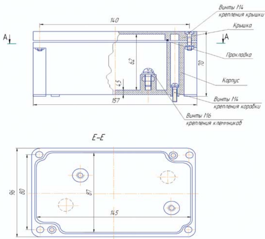
Рисунок - Габаритные и присоединительные размеры
