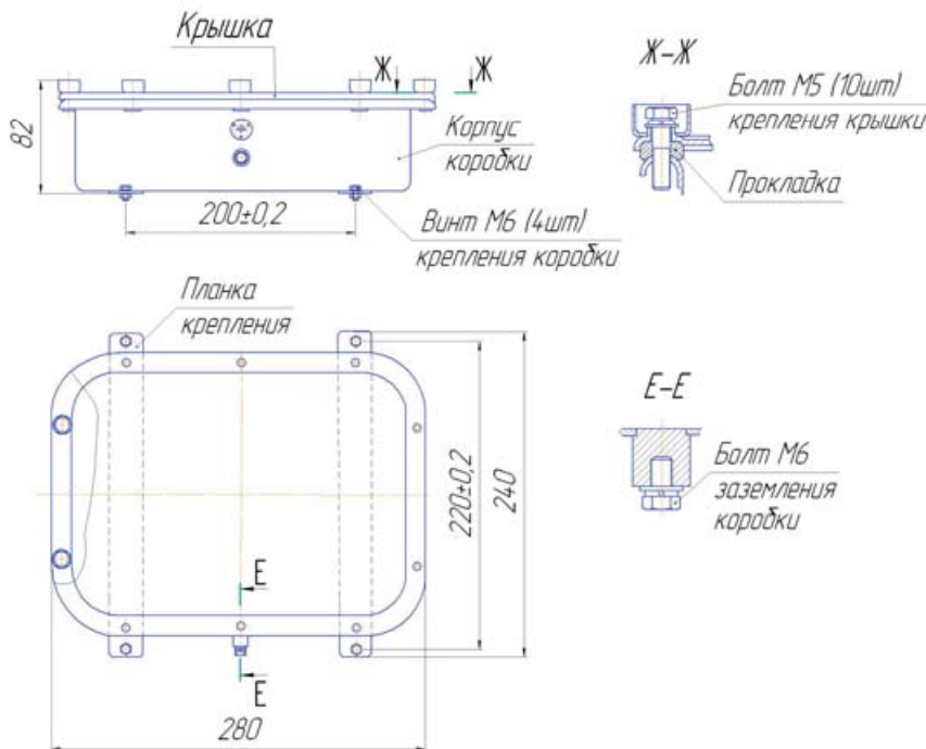
Рисунок - Габаритные и присоединительные размеры
