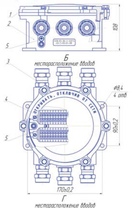
1-крышка, 2-корпус, 3-ввод кабельный, 4-клеммник, 5-знак заземления, 6-зажим заземления
